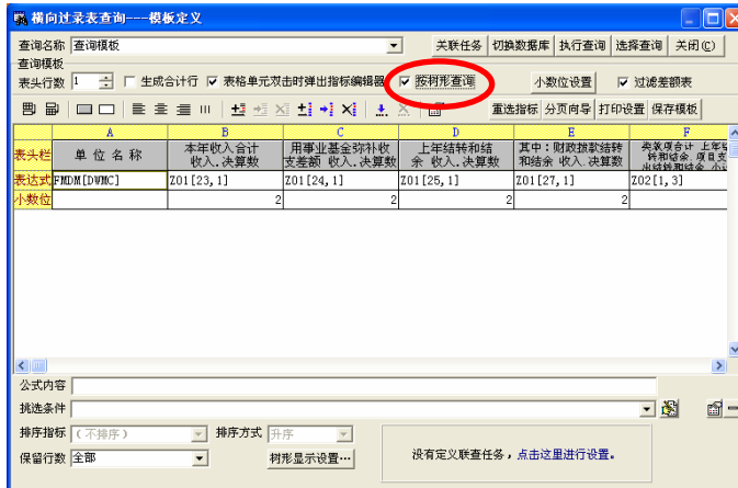
图 8.2-18 按树形查询
