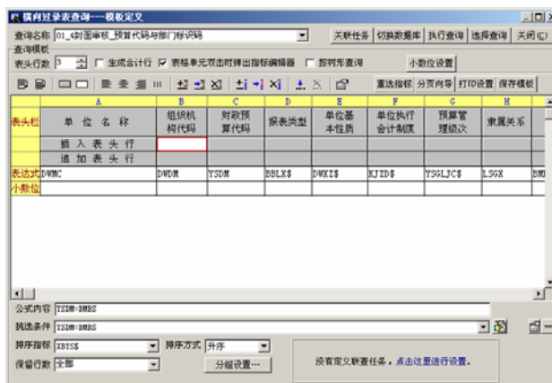
图 8.2-5 插入表头行
