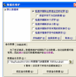
图 3.6-3 数据库维护
