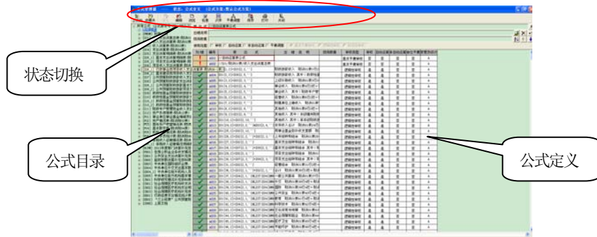
图 3.1-1 公式管理器
