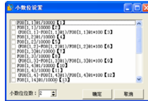
图 8.2-8 小数位设置
