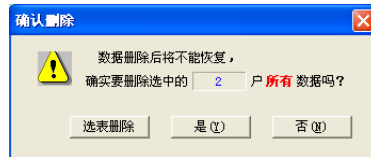
图 4.3-1 批量删除
