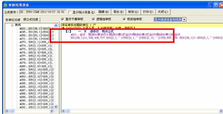
图 5.1-13 按公式过滤
