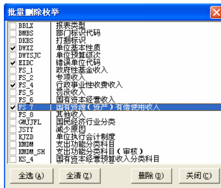
图 1.5-6 批量删除枚举字典
