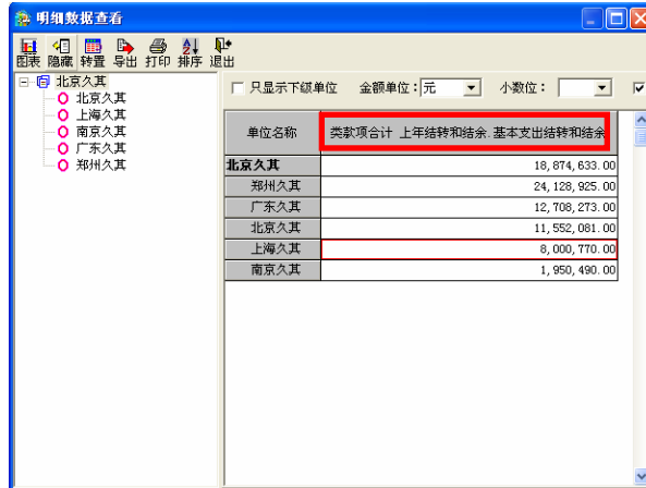
图 4.1-17 排序结果
