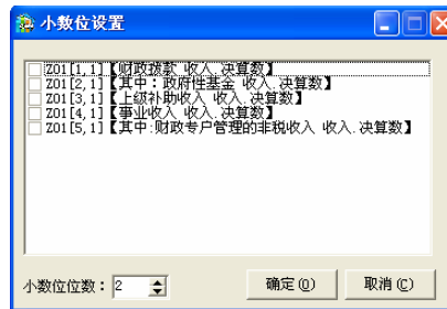
图 8.2-25 小数位设置
