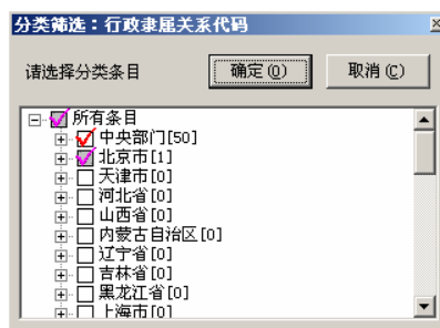
图 8.1-3 分类筛选
