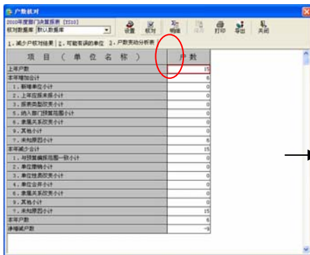
图 5.5-3 户数核对
