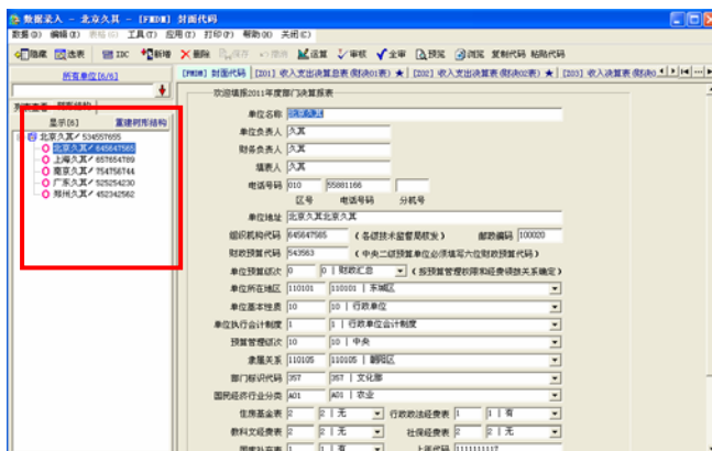
图 9.1-10 有树形结构
