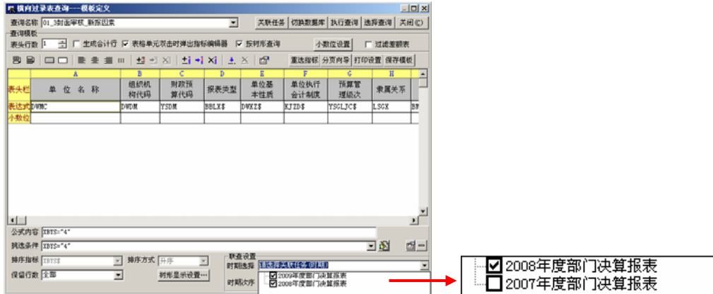
图 8.2-12 选择时期
