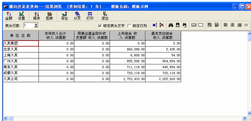
图 4.1-23 查询结果
