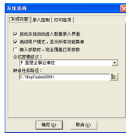
图 3.7-1 系统选项
