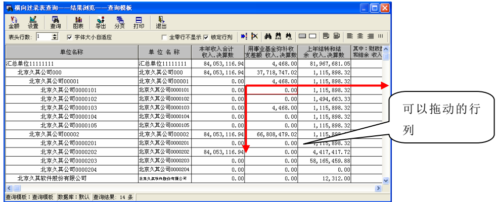
图 8.2-28 锁定行列
