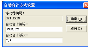
图 4.1-33 自动合计
