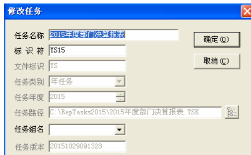
图 2.2-2 任务属性
