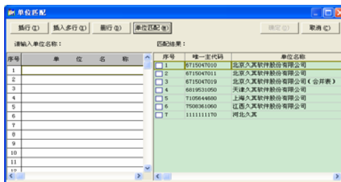
图 4.1-8 多单位匹配
