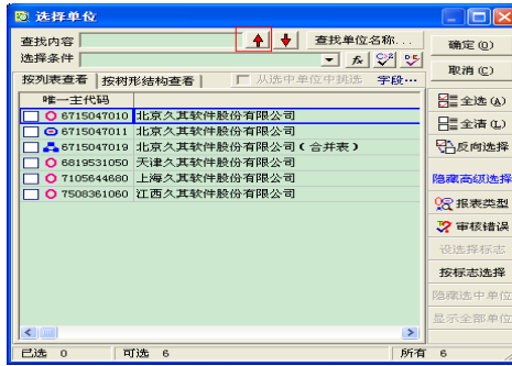
图 4.1-10 查找
