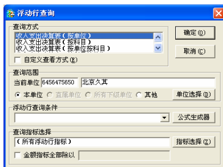
图 4.1-31 浮动行查询
