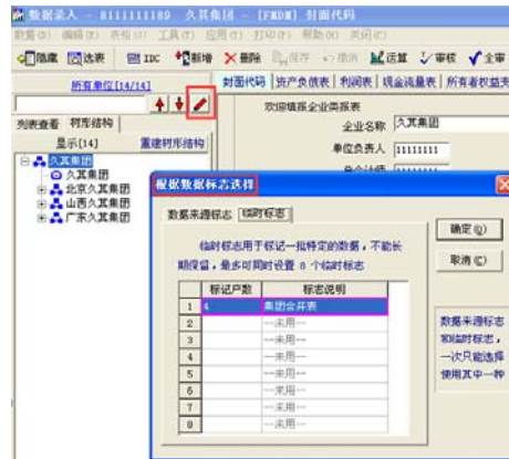
图 4.1-11 按标志选择
